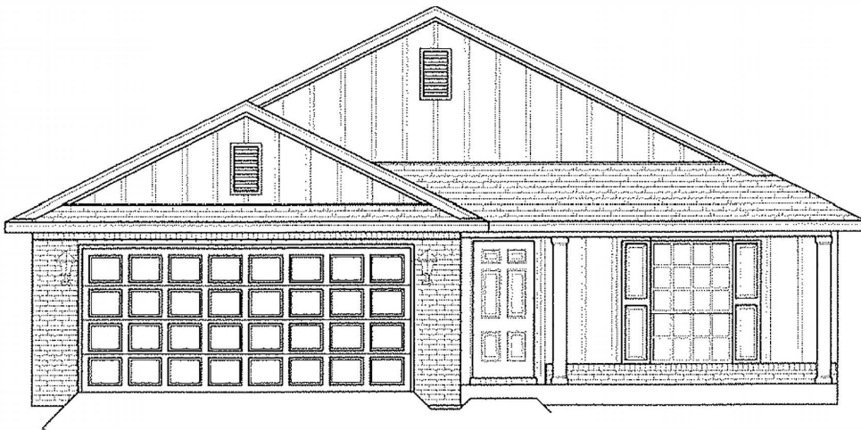
ELEVATION B
